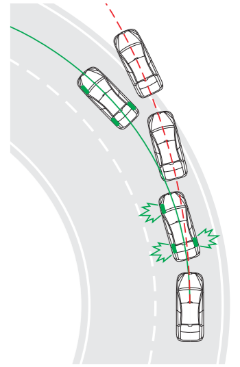
corrección de subviraje
