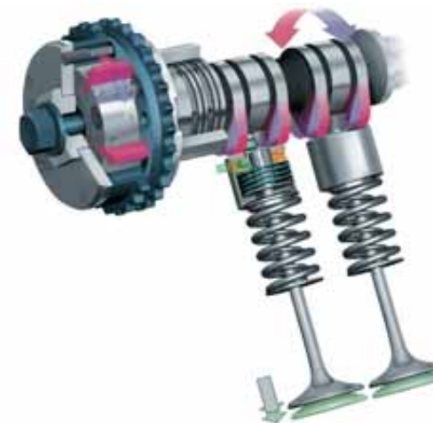
VarioCam Plus (V8 engines)
