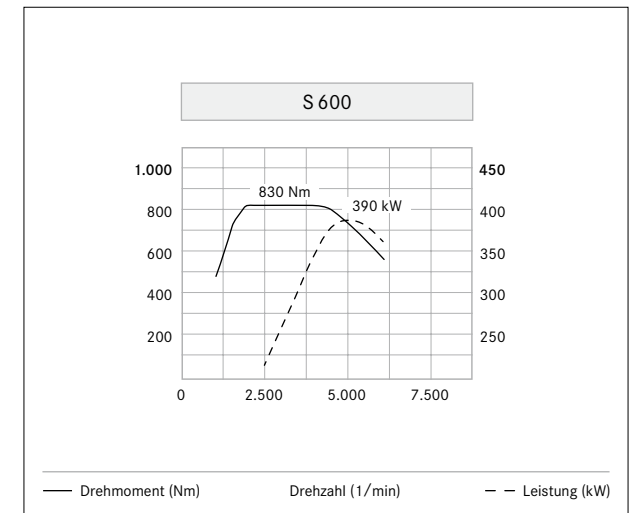
Der 12-Zylinder-Benzinmotor – höchste Kraftentfaltung, maximale Effizienz.
