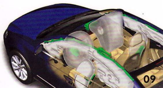
09 Air bags frontais de duplo estágio, laterais nos bancos dianteiros e cortina. O Passat conquistou nota máxima na avaliação EuroNCAP* de segurança veicular
