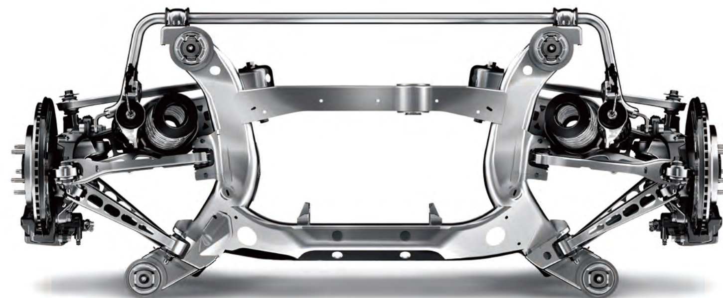
全新五连杆式独立后悬挂
