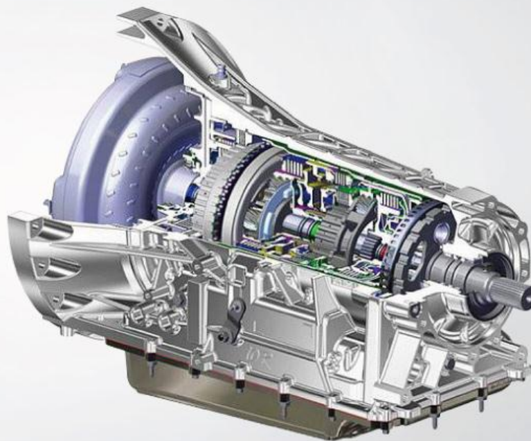
福特10速 手自一体变速器
