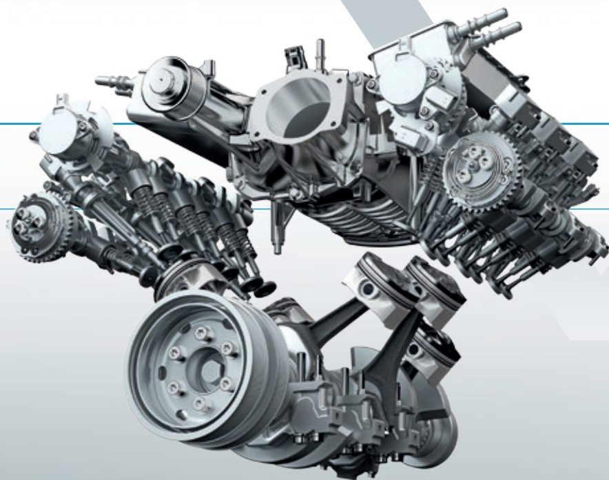
3.0升 V6 机械增压型 汽油发动机
