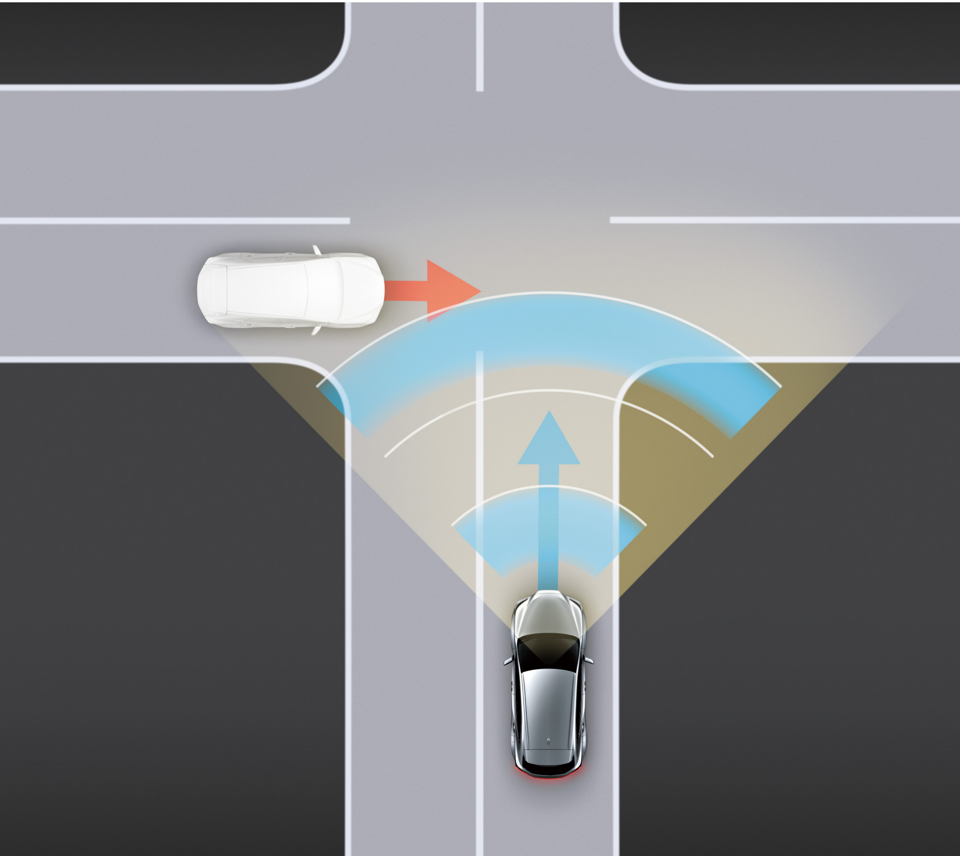
预碰撞安全系统PCS带紧急转向辅助功能ESA
