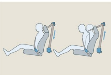
ELR 三点式安全带 (预紧限力式) 前排安全带未系报警提示
