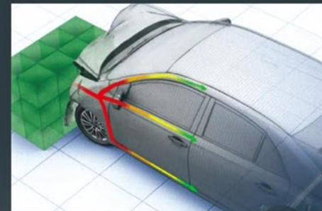
碰撞能量分散车身示意 (正面)
