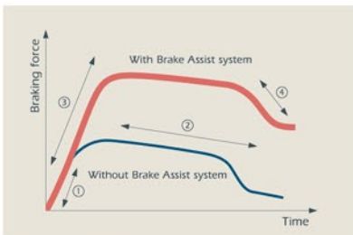
高制动性能刹车系统 BA 刹车辅助系统
