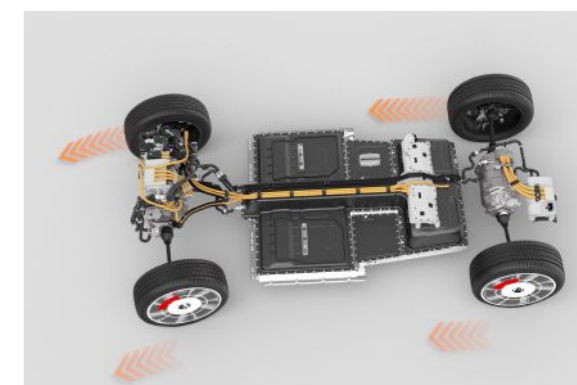
408匹全驱双电机
