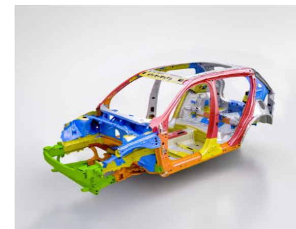
超高强度硼钢车身结构
