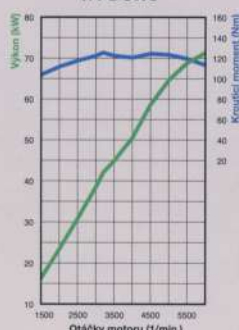
1.4 DOHC
