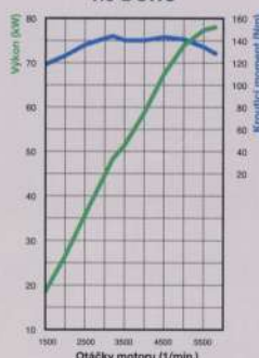
1.6 DOHC
