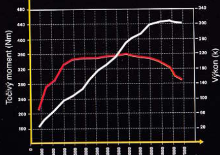
3,5 litrový benzínový šestiválec
