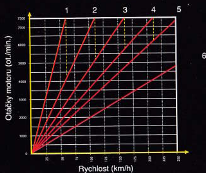
3,5 litrový benzínový šestiválec
