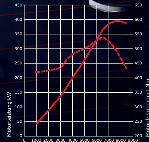
Motordrehzahl min -1 — Leistung Audi R8 V10 RWS - - - Drehmoment Audi R8 V10 RWS
