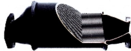
Der Drossel-Katalysator.
