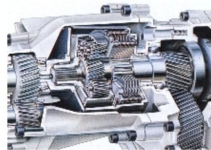
Die Lamellensperre beim Automatikgetriebe verteilt die Antriebskräfte automatisch.
