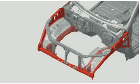
Robuster Leiterraum und RISE Sicherheitsfahrergastzelle Der Einsatz hochfester Stähle und der robuste Leiterraum erhöhen die Stabilität der RISE Sicherheitsfahrergastzelle sowie die Verwindungssteifigkeit des gesamten Fahrzeuges. Dadurch bleibt die Karosserie auch bei schwerer Zuladung und bei Gespann-Nutzung in jeder Fahrsituation stabil.
