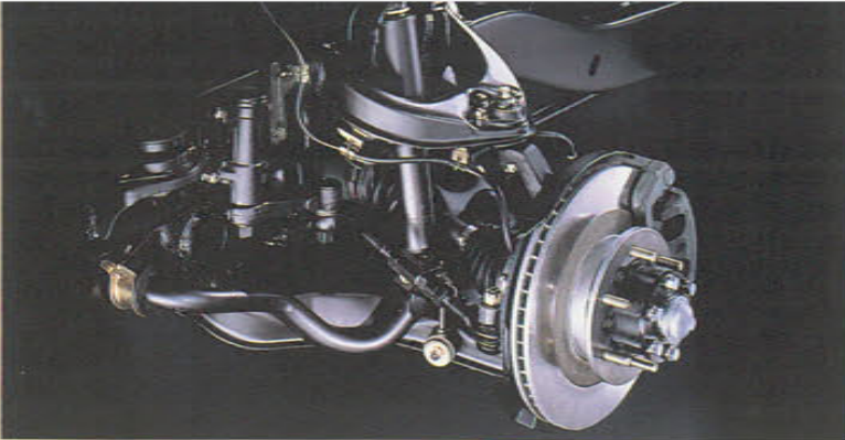
Abb.: Vorderradaufhängung 2800 TD GLS
