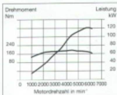
Souveräne Durchzugskraft: Der Viertakter erreicht bei 4200 min -1 sein maximales Drehmoment von 227 Nm. Im Bereich zwischen 1600 und 6400 min -1 stehen beachtliche 180 Nm zur Verfügung.
