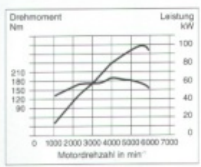
Der von System Siemens Simtec 56 elektronisch gesteuerte 16V-ECOTEC-Motor zeigt einen ausgeprägten Drehmomentverlauf, der für die leistungsfähige und komfortable Kraftentfaltung dieses modernen Motors sorgt. Das maximale Drehmoment von 185 Nm liegt bei 4000 min -1 .
