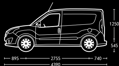
Kastenwagen mit Radstand L1 und Dachhöhe H1.
