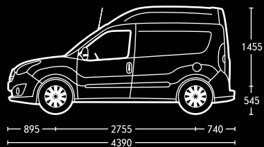
Kastenwagen mit Radstand L1 und Dachhöhe H2.
