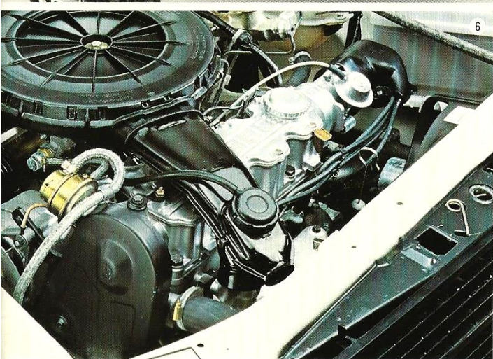
© Miniblockfeder © Federbein vorn © hydraulischer Ventilspiel-Ausgleich © Antriebseinheit © Querstromprinzip © Quer eingebauter Motor © 1.6 S-OHC-Motor
