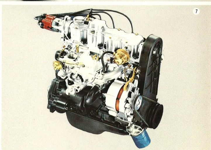
© Miniblockfeder © Federbein vorn © hydraulischer Ventilspiel-Ausgleich © Antriebseinheit © Querstromprinzip © Quer eingebauter Motor © 1.6 S-OHC-Motor
