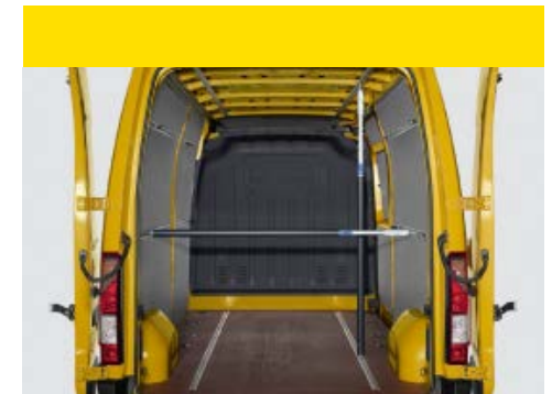
Ausziehbares Teleskopstangen 1 . Können horizontal und vertikal angebracht werden und sichern schwere Ladungen.
