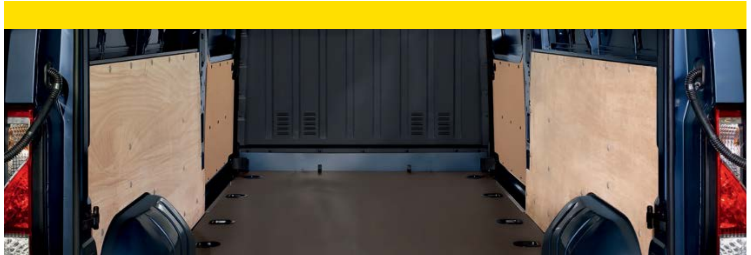
Laderaumschutz 1 . Maßgeschneiderte halb- oder vollflächige Seitenpaneele aus Holz sowie ein harzbeschichteter Holzboden schützen den Laderaum vor Beschädigung.
