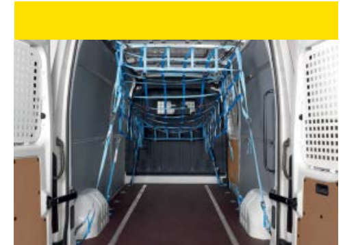
Ladungssicherungsnetz 1 . Dreidimensional und flexibel sichert das Ladungssicherungsnetz Ladungen unterschiedlicher Größen.
