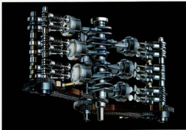
Kurbeltrieb mit Ventiltrieb
