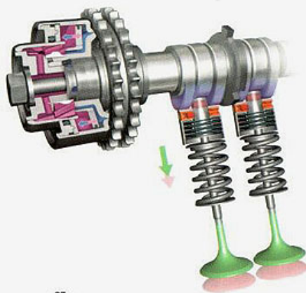
VarioCam Plus
