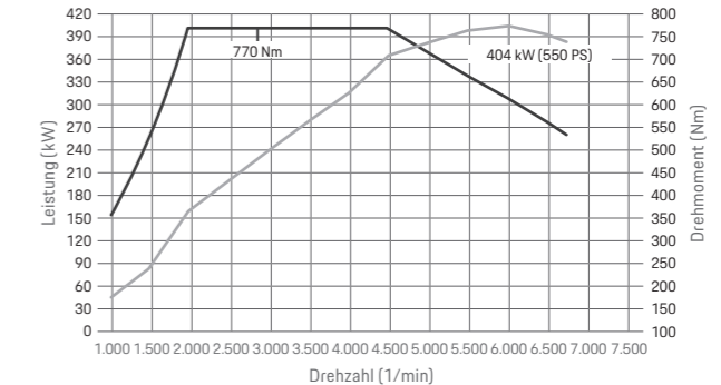
Cayenne Turbo: 404 kW (550 PS) zwischen 5.750–6.000 1/min, 770 Nm zwischen 1.960–4.500 1/min
