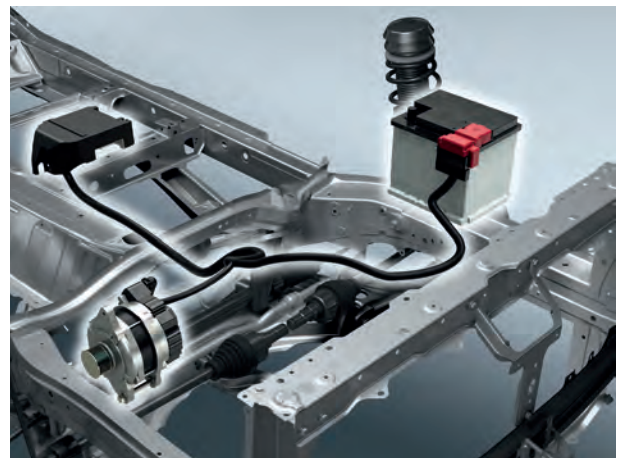
Bestandteile des SHVS Mild Hybrid Systems
