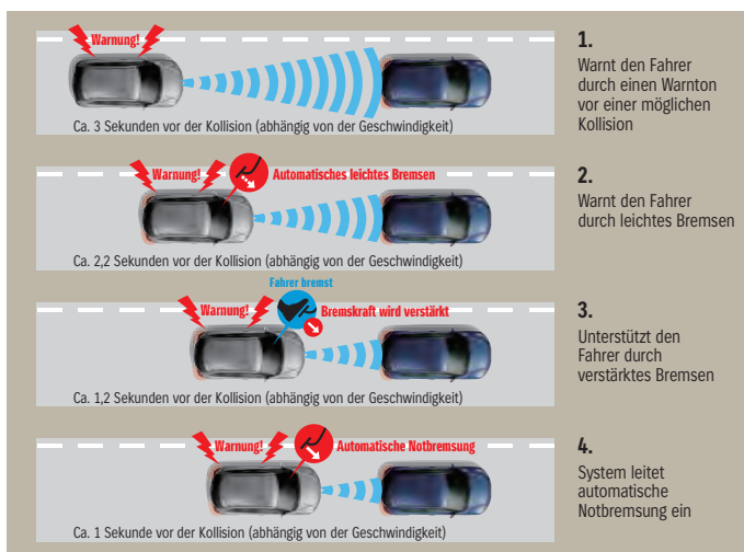
Radargestützte aktive Bremsunterstützung (RBS) 1
