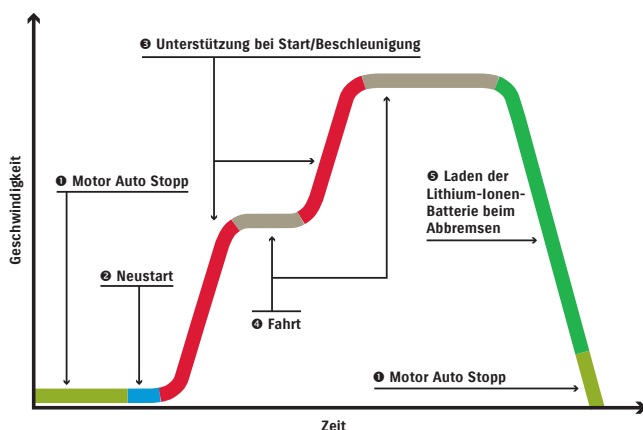
Funktionsweise des SHVS Mild Hybrid Systems
