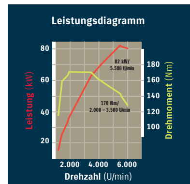
1.0-Liter-BOOSTERJET-Motor
