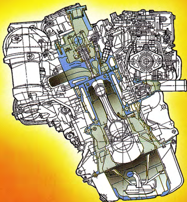
Der 2,0-l-Turbodieselmotor
