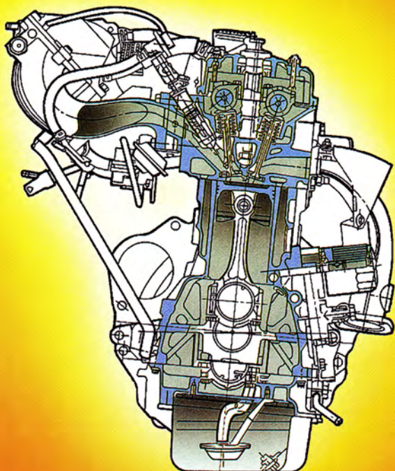
Der 1,6-l-Magermixmotor
