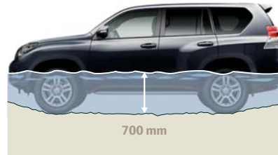
Wattiefe
