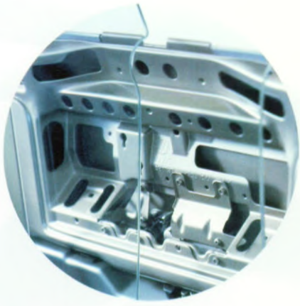
Besonders stabil: das Innenblech der Heckklappe aus Magnesium.
