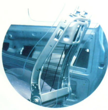
Schön leicht: Die Sitzlehngestelle werden aus Aluminium hergestellt.
