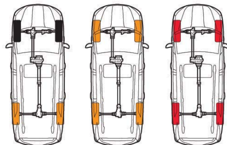
2WD Høj-gear tilstand 4WD Høj-gear tilstand 4WD Lavt-gear tilstand
