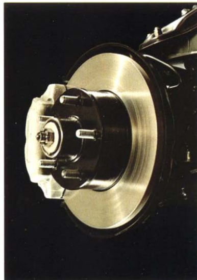
Skivbromsar fram
