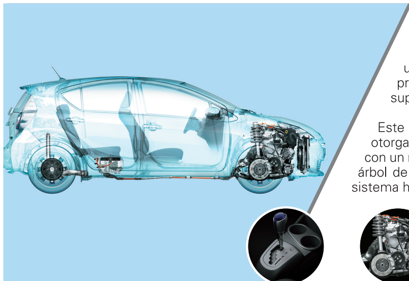
Transmisión continuamente variable controlada electrónicamente.
