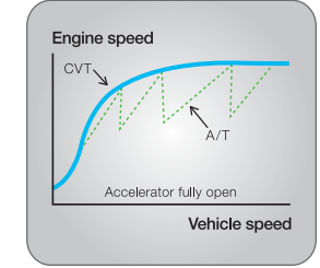
فتيس أوتوماتيك CVT CVT AT TRANSMISSION
