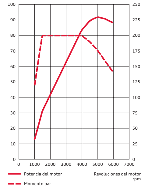
Curva de la potencia del motor 1.4 TFSI (92 kW)
