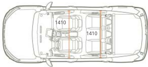
VISTA DESDE ARRIBA 5 PLAZAS
