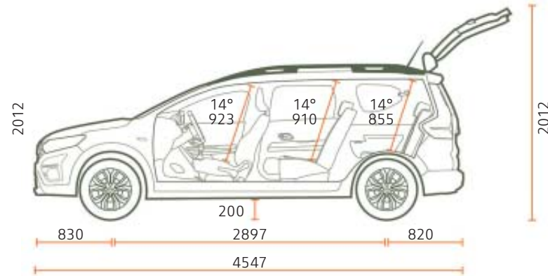
VISTA DE PERFIL DE 7 PLAZAS
