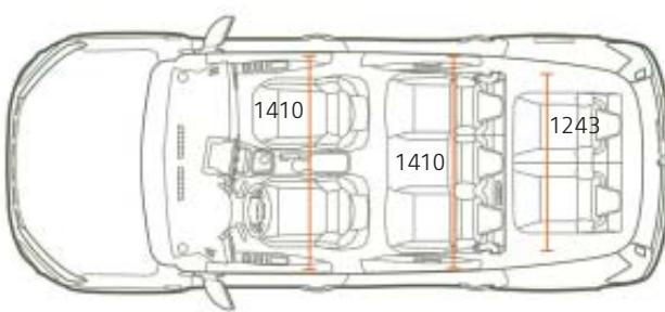
VISTA DESDE ARRIBA 7 PLAZAS
