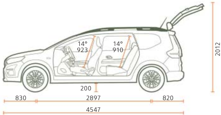
VISTA DE PERFIL 5 PLAZAS
