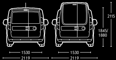
Tour con techo normal o elevado.
