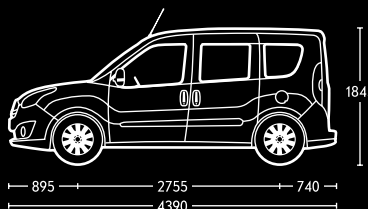
Tour con distancia entre ejes corta y techo normal.
