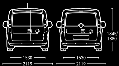
Tour con puertas traseras asimétricas o portón trasero.
