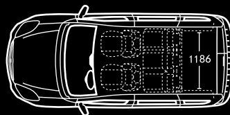
Tour con distancia entre ejes corta y 5 plazas.
