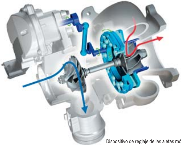
Dispositivo de reglaje de las aletas móviles
