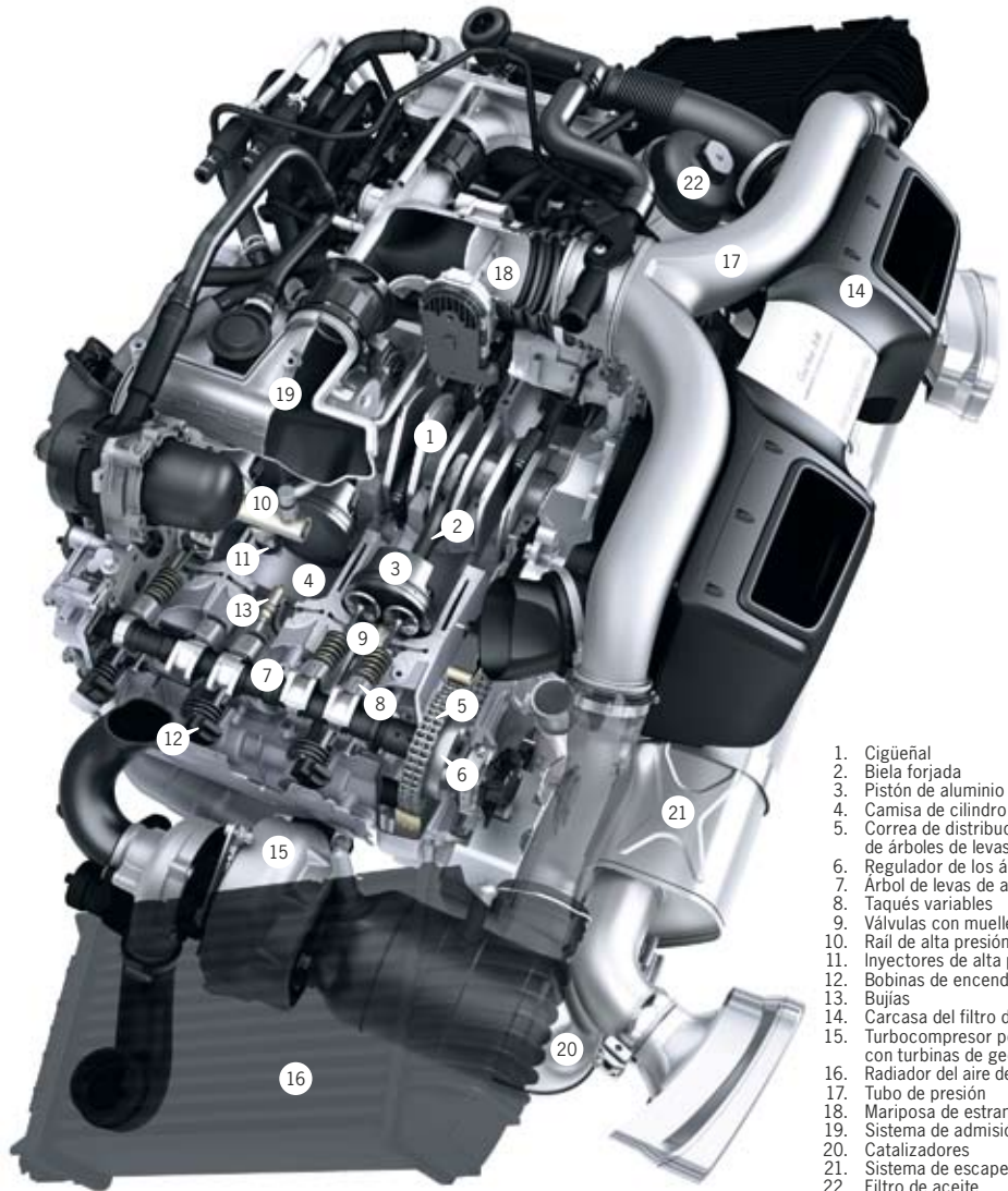
Motor con carcasa del filtro de aire de carbono visto de los nuevos modelos 911 Turbo S
