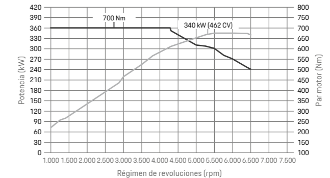
Cayenne E-Hybrid: 340 kW (462 CV) entre 5.250–6.400 rpm, 700 Nm entre 1.000–3.750 rpm
