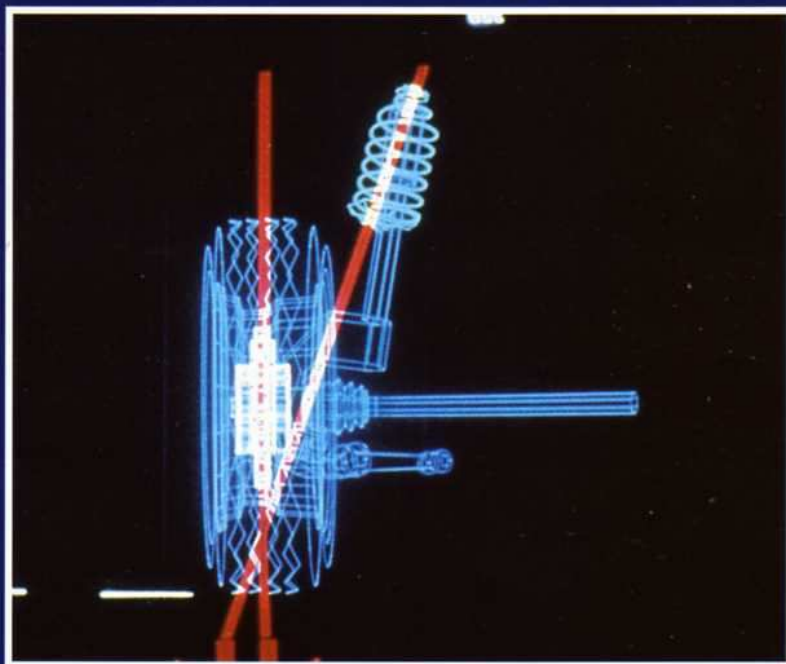
Sistema de suspensión Mc Ph con brazo a tierra negativo (
