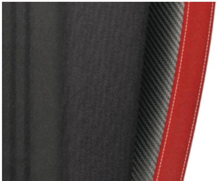
Montecarlo
