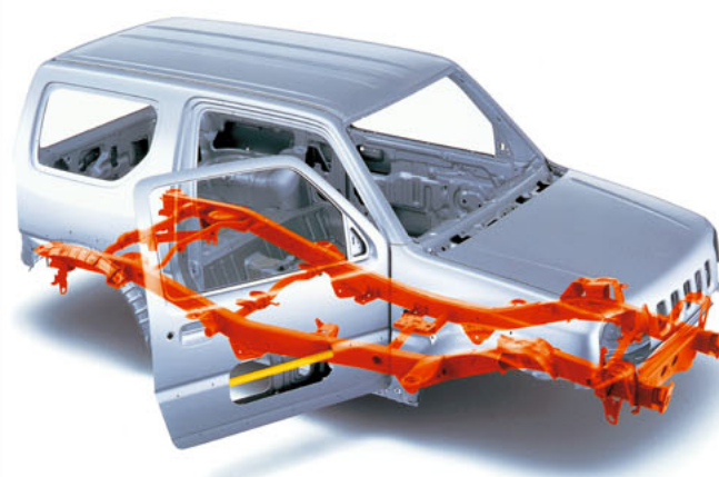
Chasis escalonado
