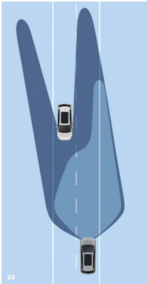
03 Kaukovalojärjestelmä Dynamic Light Assist vastaa järjestelmärajoitusten puitteissa optimaalisesta valaistuksesta pimeällä ajettaessa. Vastaan tulevan liikenteen aikana järjestelmä himmentää valaistusta osittain, jolloin ajorata pysyy edelleen hyvin valaistuna. L
