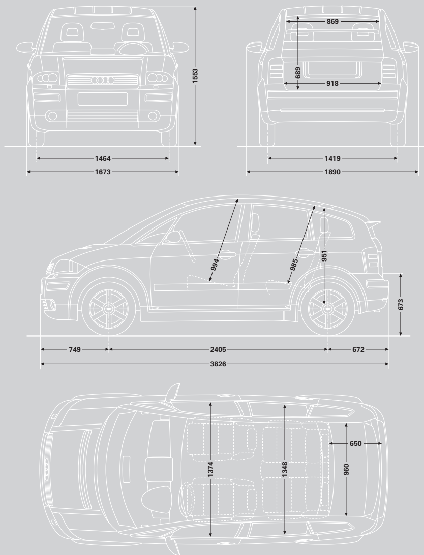
Dimensions en millimètres.
