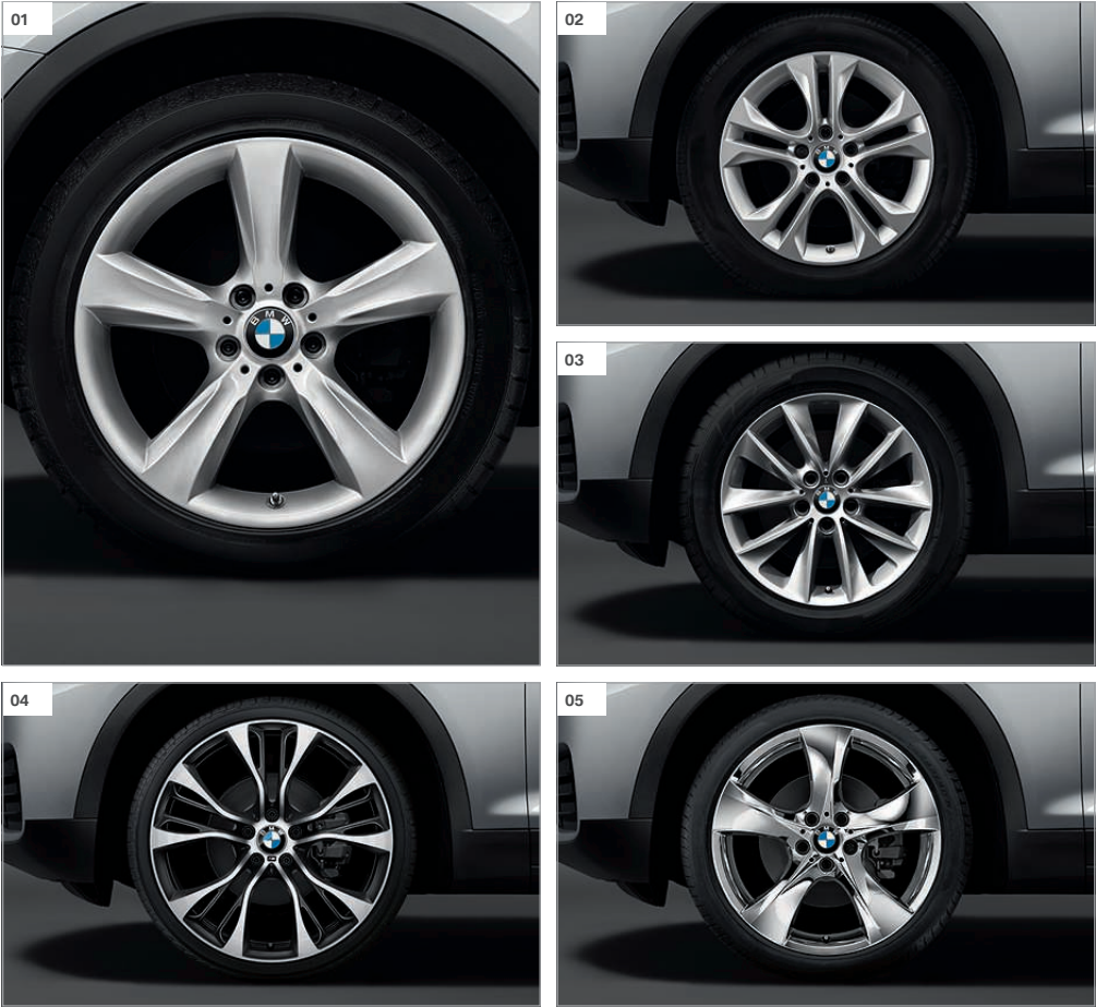
[ 01 ] Jantes en alliage léger 19" (48 cm) style 606 à rayons en étoile avec monte pneumatique mixte. Dimensions : 8,5 J x R 19 à l'avant, pneumatiques 245/45 R 19 ; 9,5 J x R 19 à l'arrière, pneumatiques 275/40 R 19. [ 02 ] Jantes en alliage léger 18" (46 cm) style 605 à rayons doubles, 8 J x 18, pneumatiques 245/50 R 18. [ 03 ] Jantes en alliage léger 18" (46 cm) style 307 à rayons en V, 8 J x 18, pneumatiques 245/50 R 18. [ 04 ] Jantes en alliage léger 21" (53 cm) BMW M Performance style 599 M à rayons doubles, noir mat, bicolores et forgées, polies du côté visible, avec logo M quatre couleurs et monte pneumatique mixte. Dimensions : 8,5 J x 21 à l'avant, pneumatiques 245/35 R 21 ; 10 J x 21 à l'arrière, pneumatiques 275/30 R 21. [ 05 ] Jantes en alliage léger 20" (51 cm) style 311 à rayons en étoile, chromées, avec monte pneumatique mixte. Dimensions : 8,5 J x 20 à l'avant, pneumatiques 245/40 R 20 ; 10 J x 20 à l'arrière, pneumatiques 275/35 R 20.
