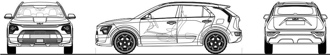
Dimensions Niro EV 100 % électrique (mm)
