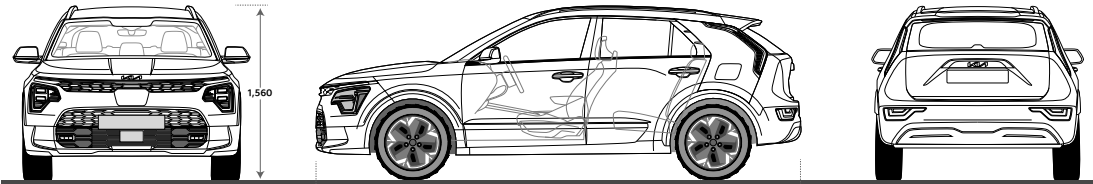
Dimensions Niro EV 100 % électrique (mm)
