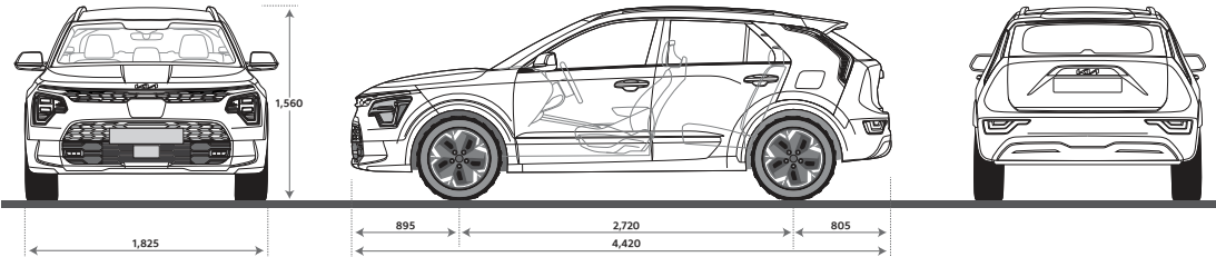
Dimensions Niro EV 100 % électrique (mm)
