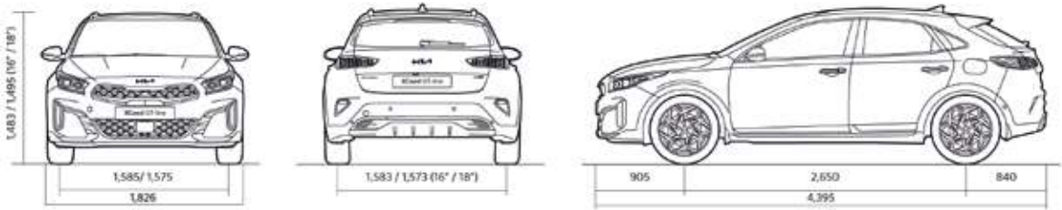
Dimensions versions Thermiques (mm)
