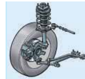
Train avant de type pseudo Mac Pherson : une précision optimale du guidage dans les courbes.
