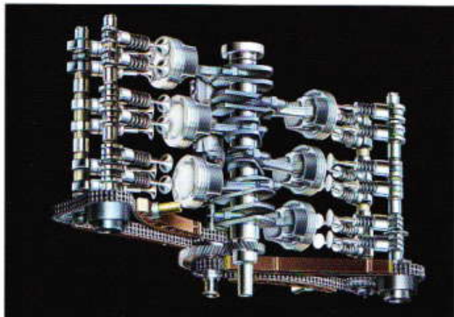
Viebrequin avec soupapes
