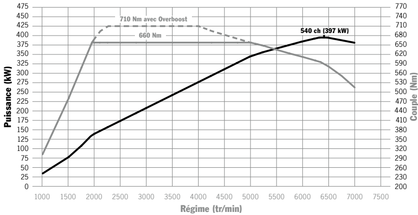
911 Turbo et 911 Turbo Cabriolet : 660 Nm entre 1 950 et 5 000 tr/min (avec Overboost : 710 Nm entre 2 250 et 4 000 tr/min), 540 ch (397 kW) à 6 400 tr/min
