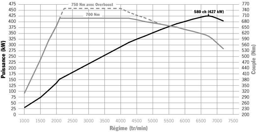
911 Turbo S et 911 Turbo S Cabriolet : 700 Nm entre 2 100 et 4 250 tr/min (avec Overboost : 750 Nm entre 2 250 et 4 000 tr/min), 580 ch (427 kW) à 6 750 tr/min
