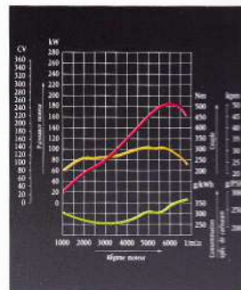
Un harmonieux développement de la courbe de puissance
