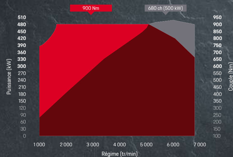
Cayenne Turbo S E-Hybrid : 680 ch (500 kW) entre 5 750 et 6 000 tr/min, 900 Nm entre 1 500 et 5 000 tr/min
