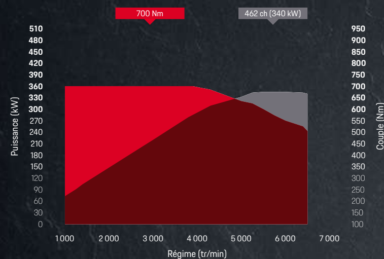
Cayenne E-Hybrid : 462 ch (340 kW) entre 5 250 et 6 400 tr/min, 700 Nm entre 1 000 et 3 750 tr/min
